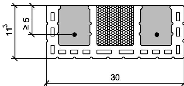
Betonquerschnitt ≥ 70 cm 2
