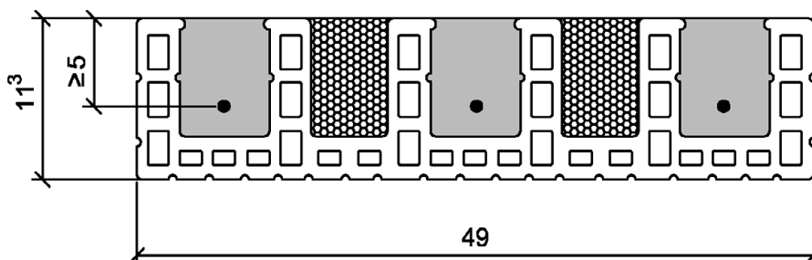
Betonquerschnitt ≥ 125 cm 2
