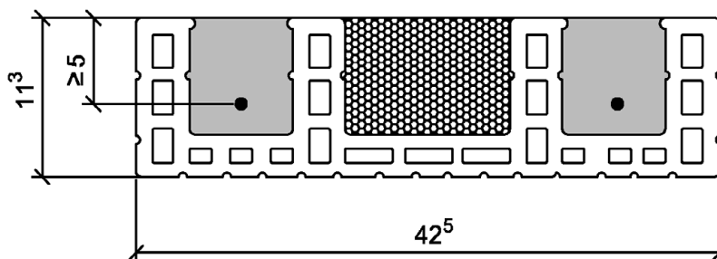
Betonquerschnitt ≥ 125 cm 2
