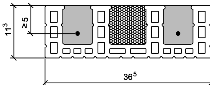
Betonquerschnitt ≥ 85 cm 2
